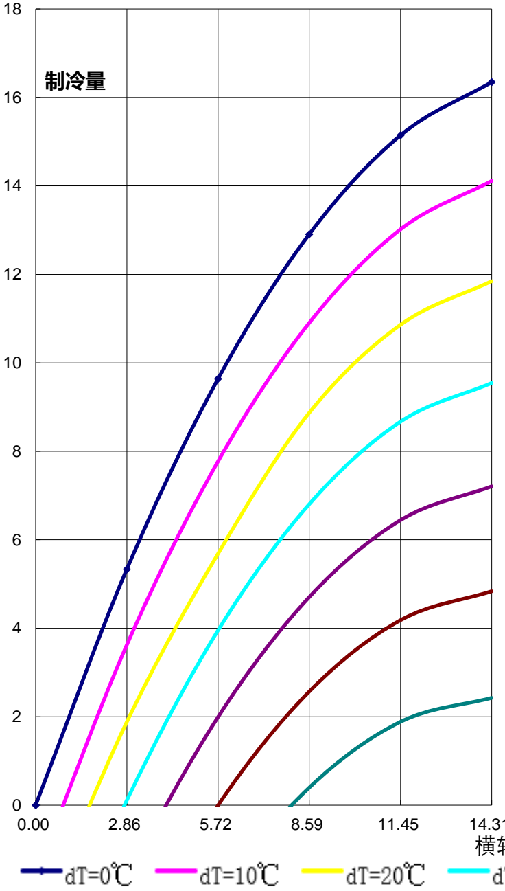
制冷量/电流曲线
